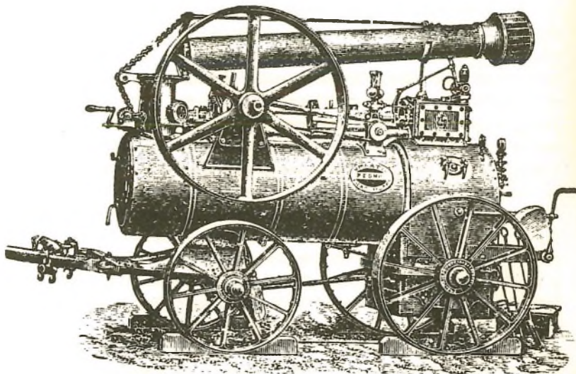
Umrathe-féle lokomobil
