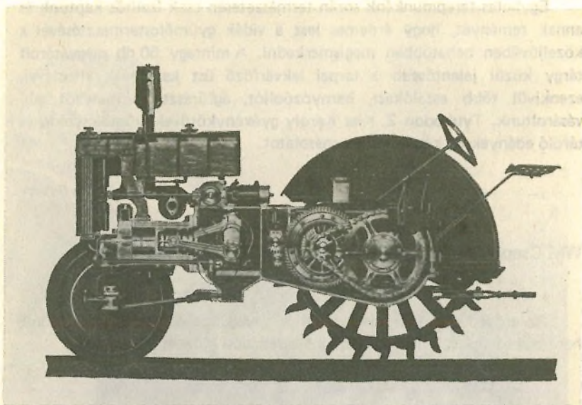
A „Csepel” traktor hosszmetsete
