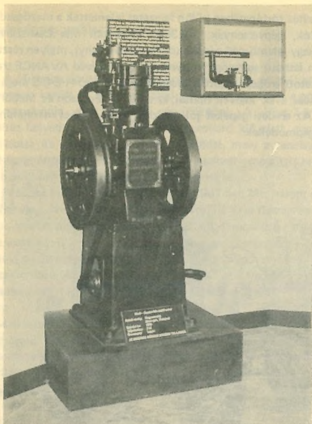
Bánki—Csonka féle stabil motor (1898)
