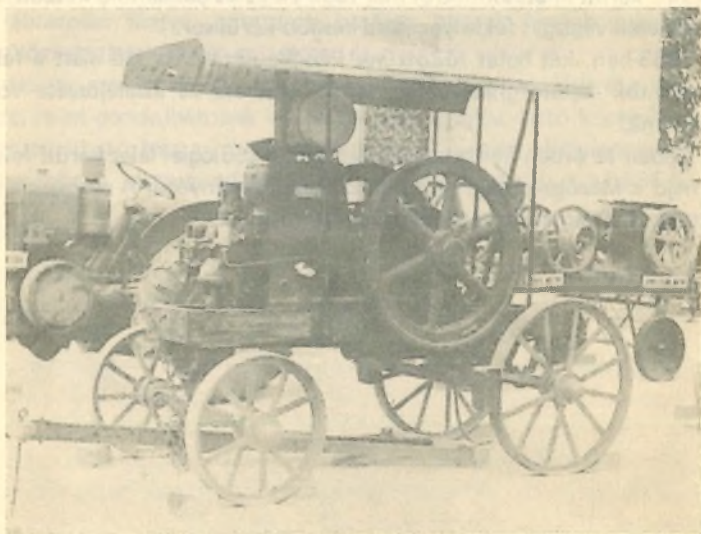
H-S-C-S benzinüzemű lokomobil (1912)
