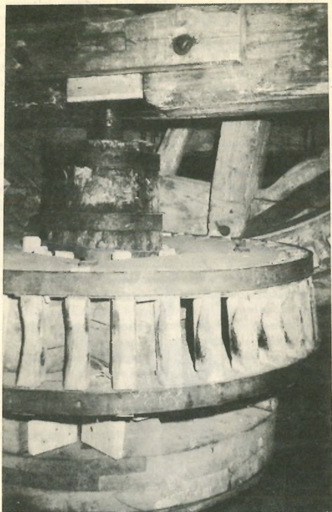
A szélmalom erőátviteli szerkezete
